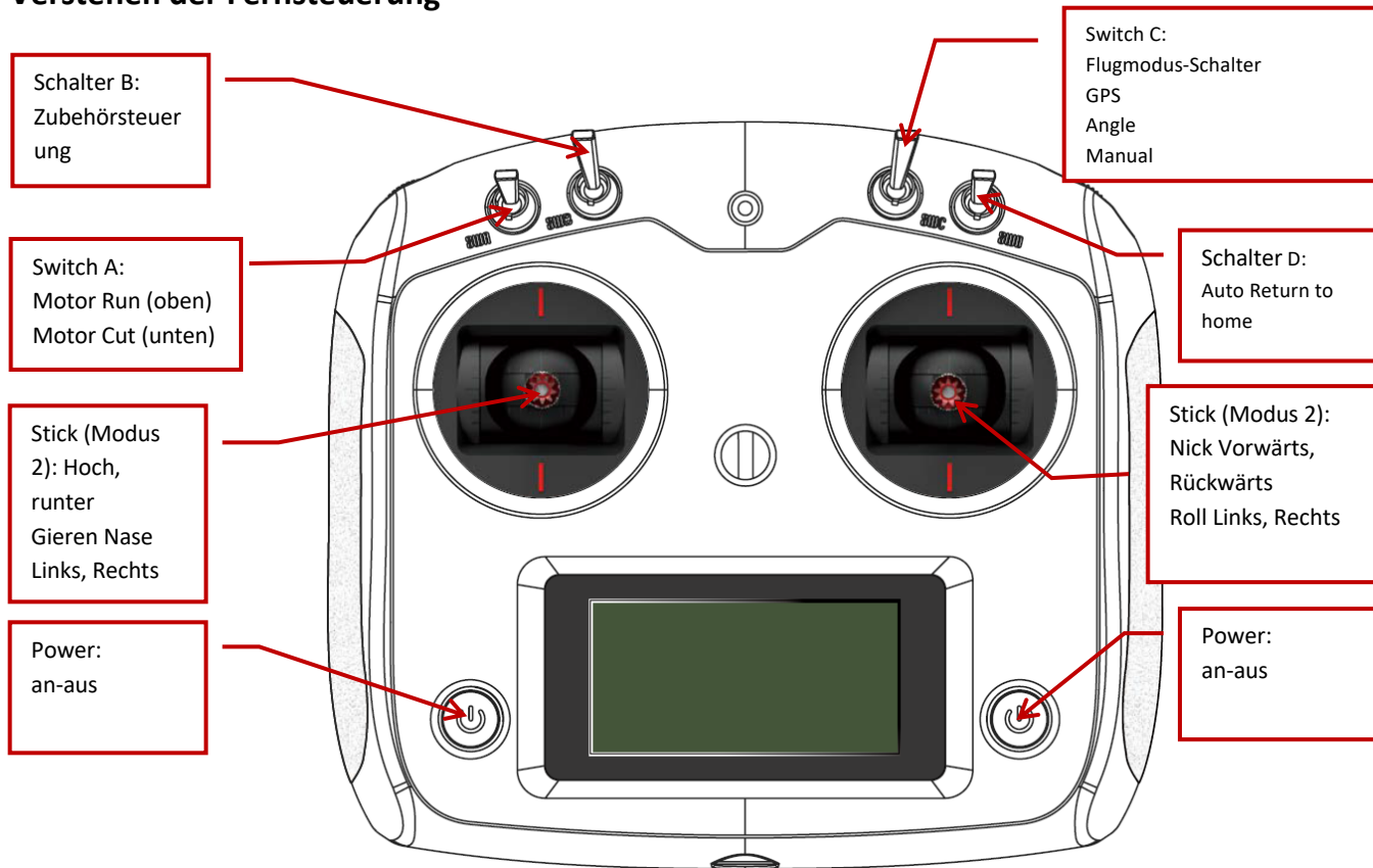
Fig. 2 Vorderseite der Fernsteuerung
