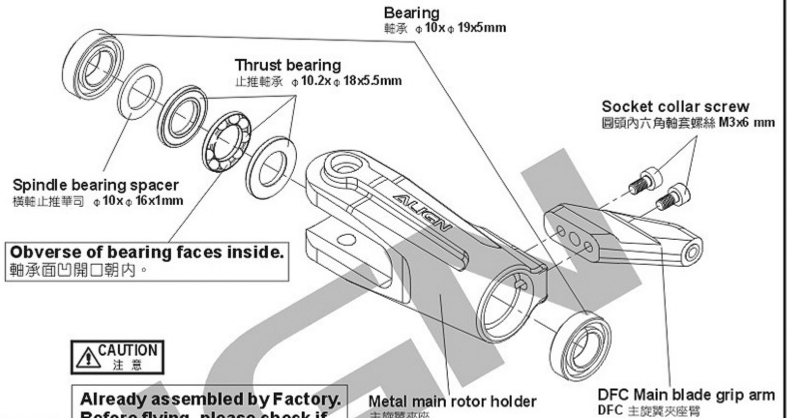
Metal main rotor holder 金屬主旋翼夾座
