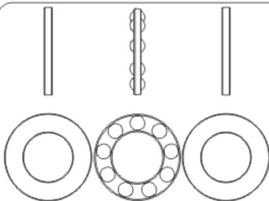
Thrust bearing 止推軸承(φ10.2xφ18x5.5mm) x 2
