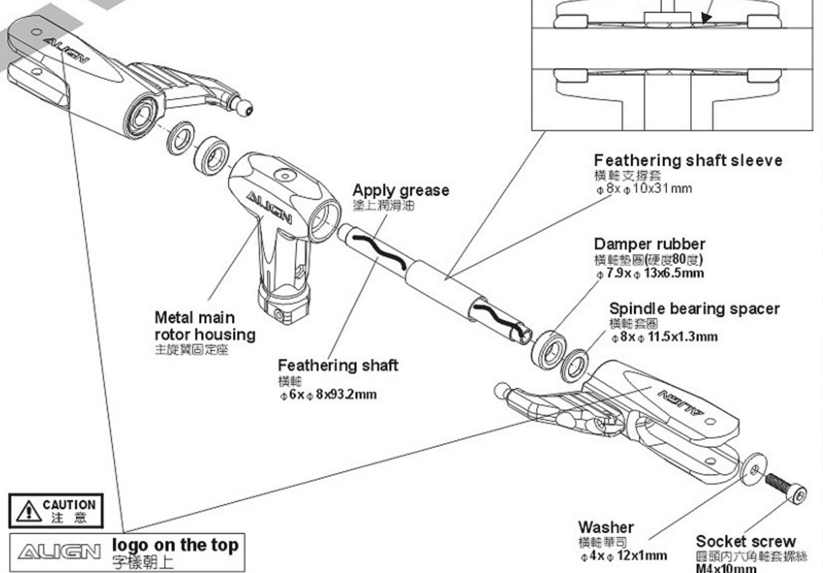
Damper rubber-black 80° 橫軸墊圈 黑色80° (φ7.9xφ13x6.5mm) x2
