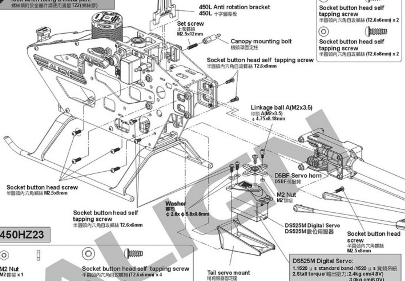
Linkage ball A(M2x3.5) 球頭 A(M2x3.5) ( \phi 4.75 \times 8.18 \text{mm} ) x1
