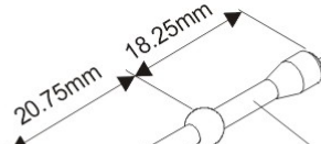
Flybar control rod 平衡翼控制球桿 φ 4.3X39mm
